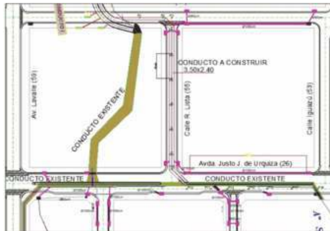
ANTEPROYECTO HIDRÁULICO DE LA CUENCA BAJA DEL ARROYO SAN MARTIN PROPUESTO POR EL EQUIPO TÉCNICO DE LA MUNICIPALIDAD DE POSADAS
