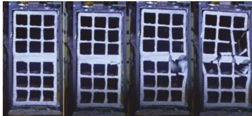
Figura 1. Secuencia de falla en una celda de mampostería
